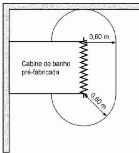
Figura 19 — Cabine de banho pré-fabricada
