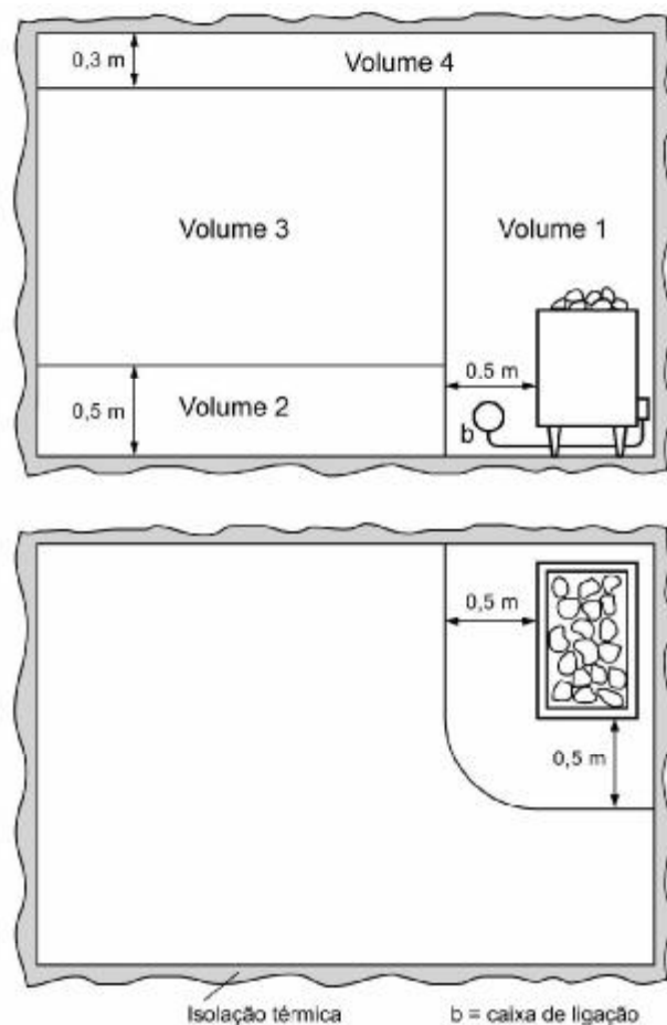
Figura 22 — Volumes de uma sauna
