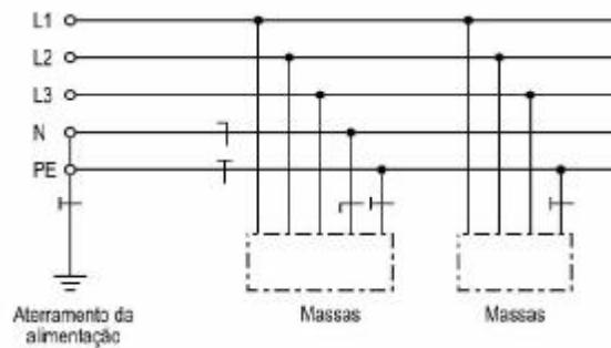
Figura 1 — Esquema TN-S
