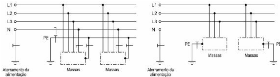
Figura 4 — Esquema TT
